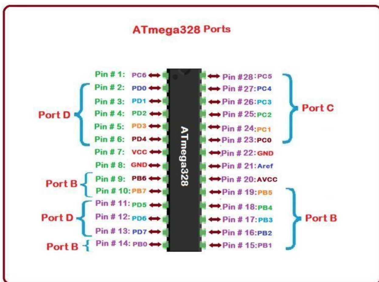
Fig 2 ATmega 328 port
