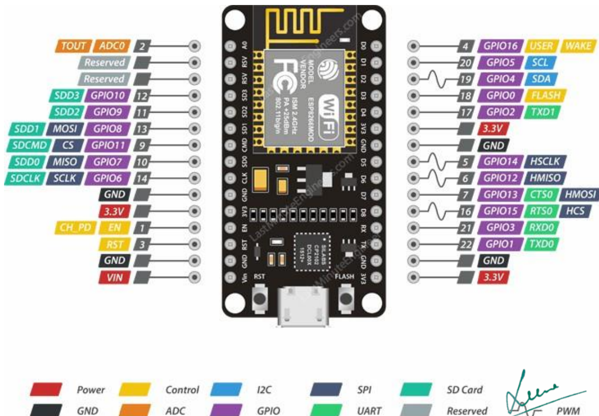
Fig 9 Node mcu
